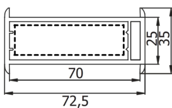
Statik-Kopplung Basis 70 7053 90-227-10 Stahl
