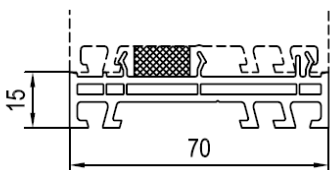
15 mm Nr. 140209
