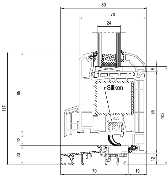
4000 – Nebeneingangstür – Aluminiumbodenschwelle
