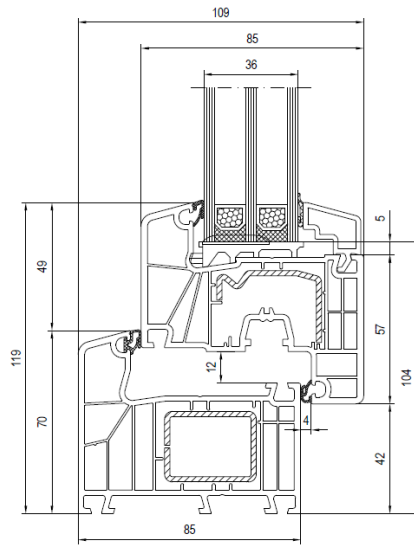
Blendrahmen Nr. 170x02 – Flügel Nr. 170x20
