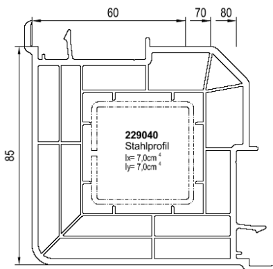
Kopplung Nr. 140248 Stahlprofil Nr. 229040
