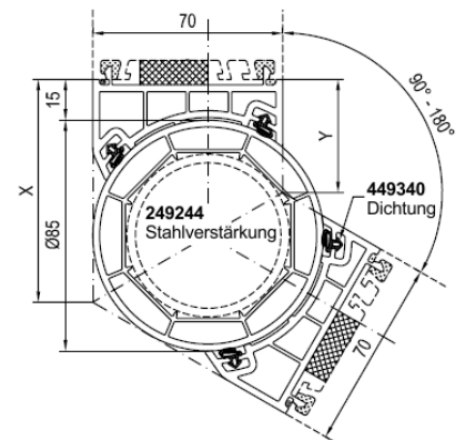
Kopplung Nr. 140244 Adapter Nr. 140243
