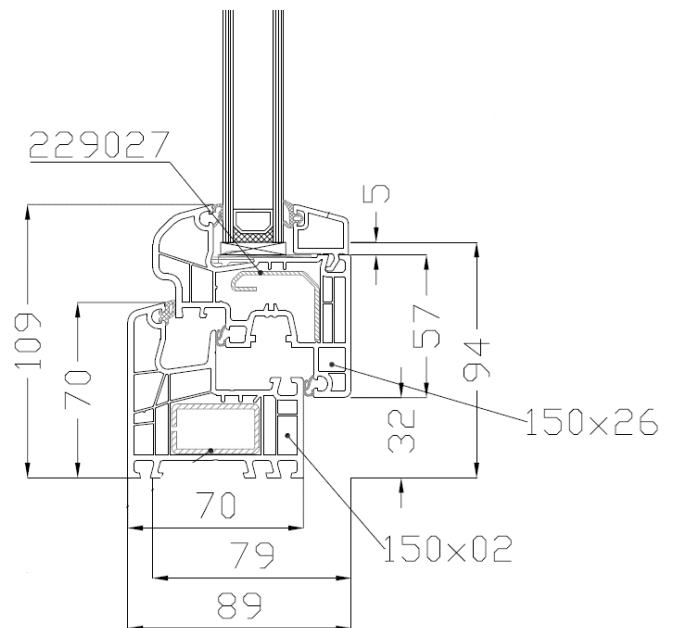
5000 Plus – Dreh-Kipp – DK
