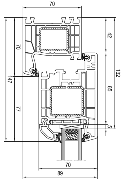
Blendrahmen Nr. 140x02 – Flügel Nr. 140x31
