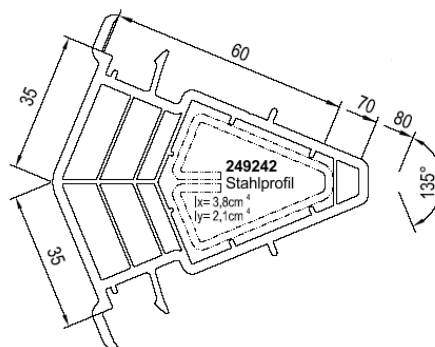
Kopplung Nr. 140249 Stahlprofil Nr. 249242
