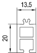
FBA Nr. 120106
