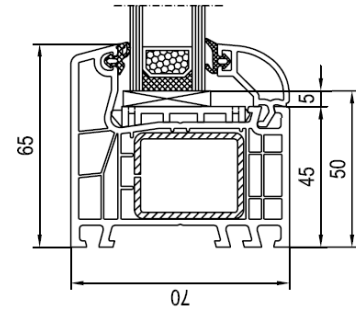
Blendrahmen Nr. 140x01
