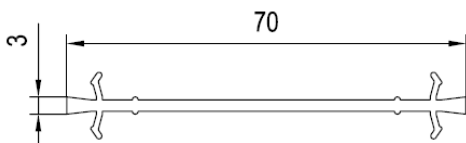
Kopplung Nr. 140203
