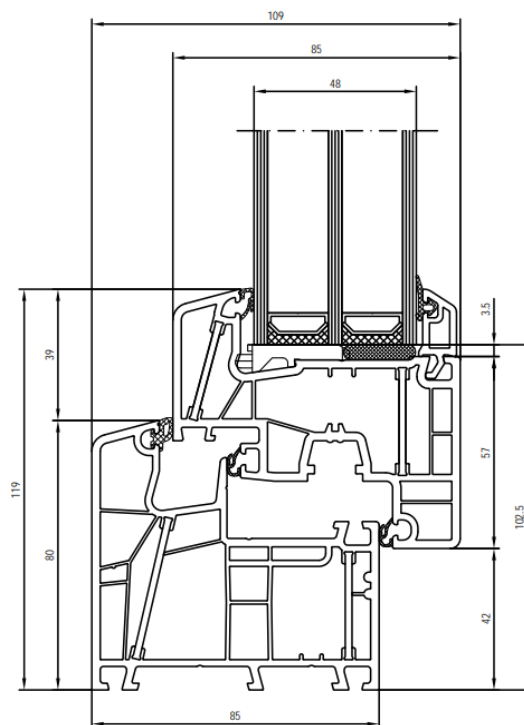
Blendrahmen Nr. 080004 – Flügel Nr. 080020
