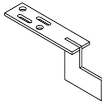
Montageanker Nr. 622332
