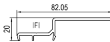
Kastenanschlussprofil Nr. 144233
