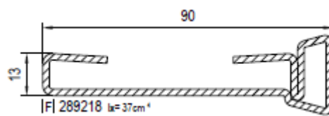
Stahlprofil Nr. 289218
