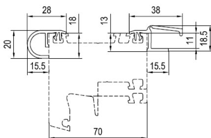
Anschlussituation
