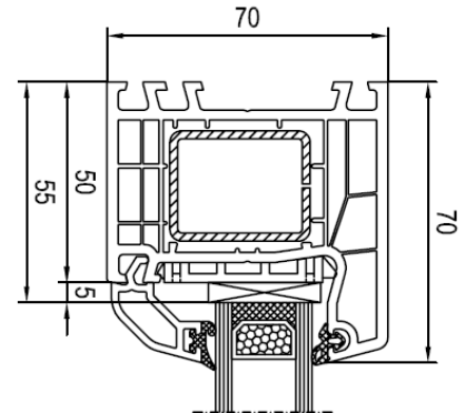
4000 – Nebeneingangstür Festverglasung
