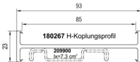
Kopplung Nr. 180267 Stahlprofil Nr. 209900
