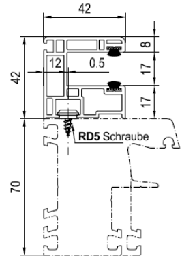
Rastkopfschraube Nr. RD5
