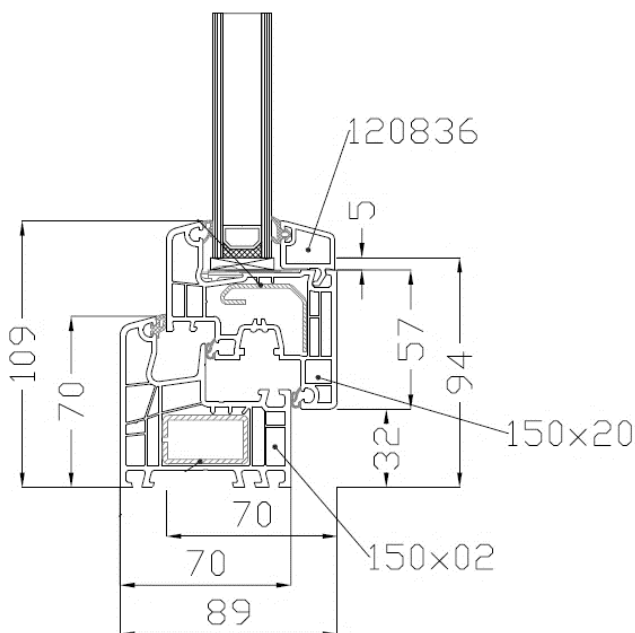
Blendrahmen Nr. 150x02 – Flügel Nr. 150x20
