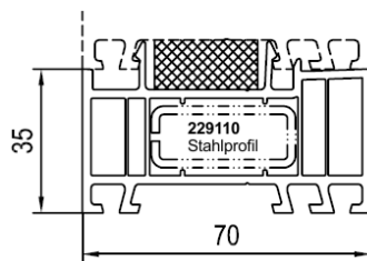
35 mm Nr. 140205
