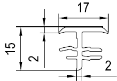
Kopplung Nr. 120224
