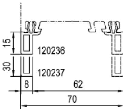
Anschlussituation 15 mm und 30 mm
