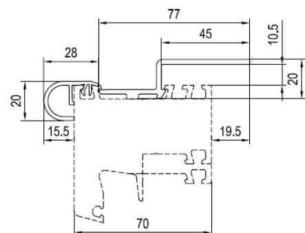
Anschlussituation
