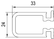
Abdeckung Nr. 120219
