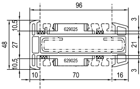
Kopplung Nr. 140218 Stahlprofil Nr. 229018
