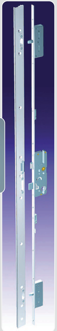
Dreipunktverriegelung mit Schließteil
